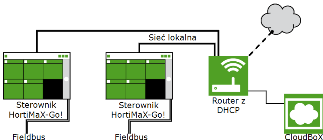
Rysunek 1-1: Schemat połączenia sieciowego
